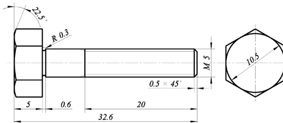
10. Zavrtanj M5
